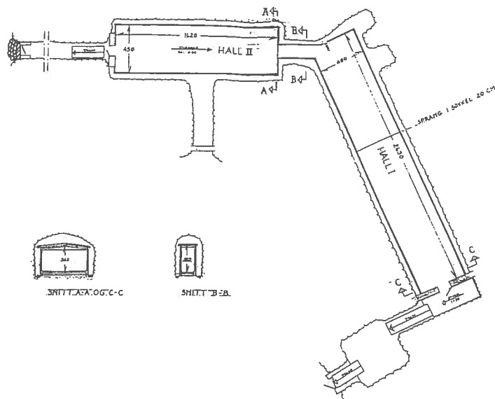
Snittegning av anlegget i Mokollen. Tegning utlånt fra Jon Vegar Haugåsen.
